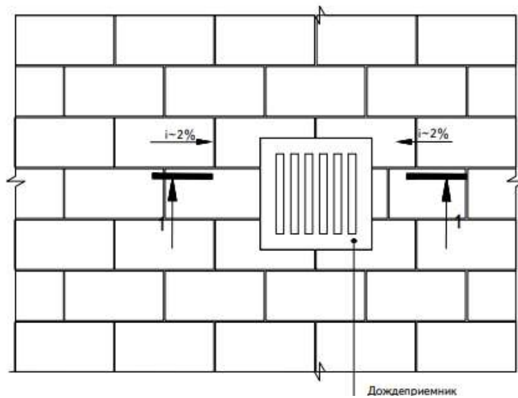
Илл. 1.2.14. ПРИНЦИПАЛЬНАЯ СХЕМА УСТРОЙСТВА ДОЖДЕПРИЕМНИКА НА ТРОТУАРЕ
